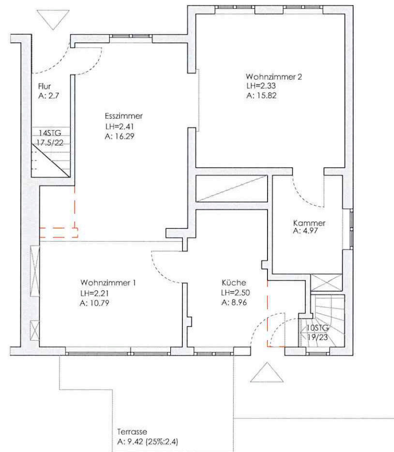
ERDGESCHOSS Kein verformungsgerechtes Aufmass, keine Wand-/Deckendickenbestimmung
