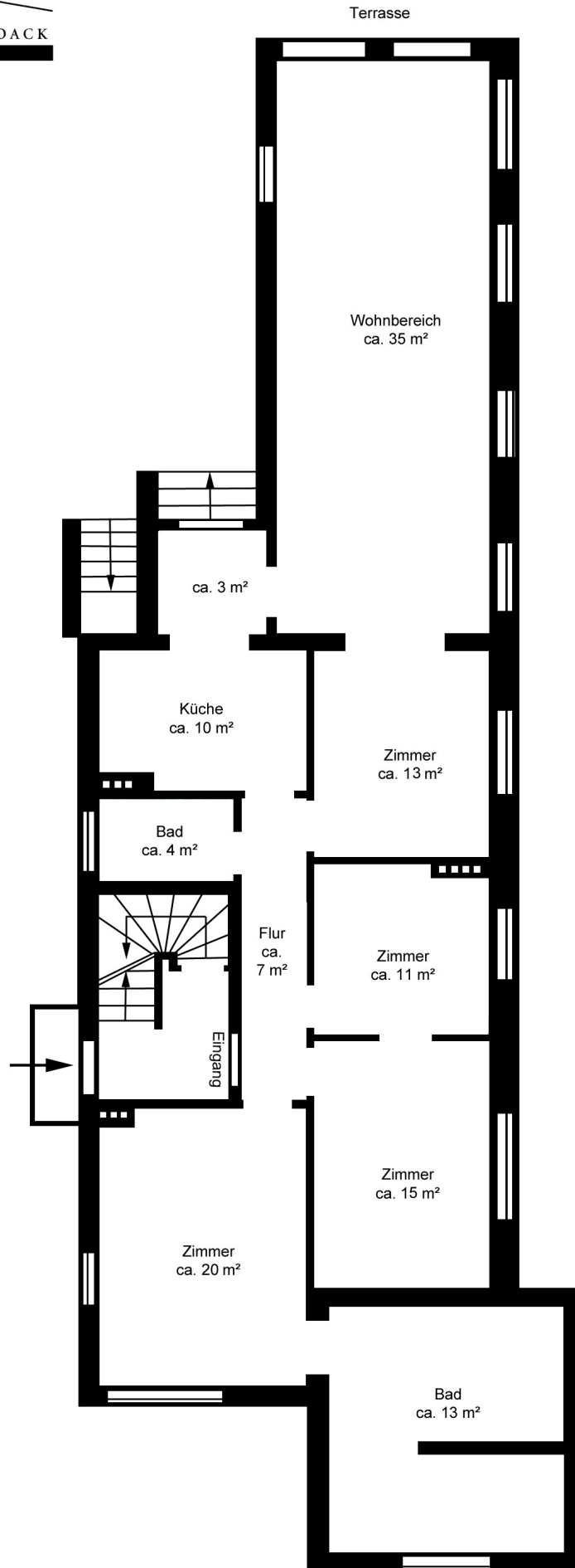
Grundriss Erdgeschoss
